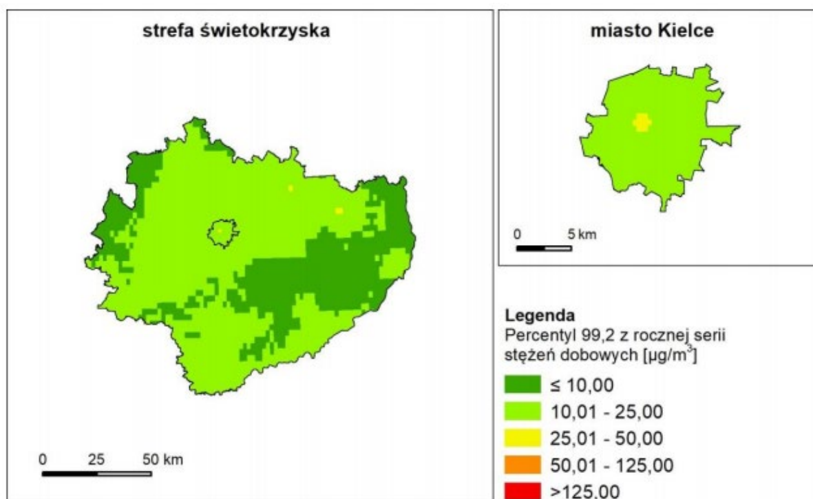
Rysunek 3: Klasyfikacja stężeń \text{SO}_x za rok 2018 (źródło: Roczna ocena jakości powietrza w województwie świętokrzyskim. Raport wojewódzki za rok 2018)
